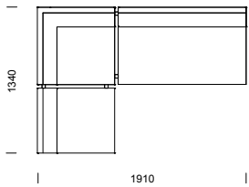
1H2 vinkelhörn utan armstöd
