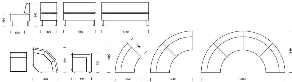
CRICKET ritningar för kombinationer – se sidan 98–99.
