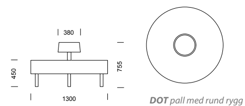
DOT pall med rund rygg
