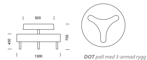
DOT pall med 3-armad rygg
