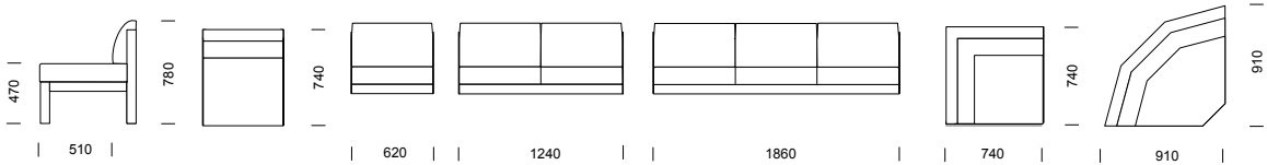
SKATE ritningar för kombinationer – se sidan 101.
