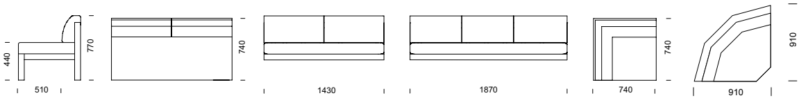
POKER ritningar för kombinationer – se sidan 100.
